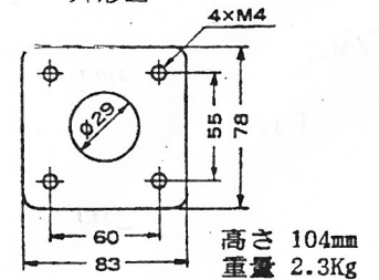
外形図
